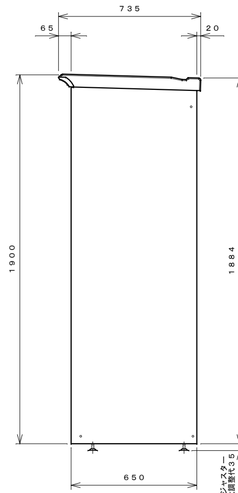
右側面図
