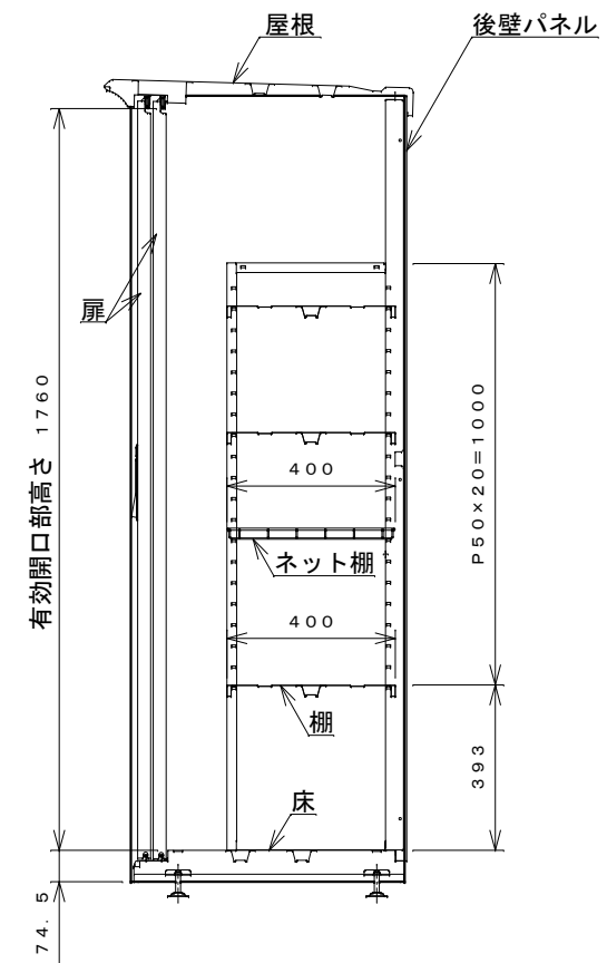
側面断面図
