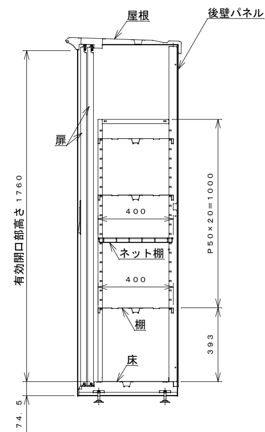
側面断面図
