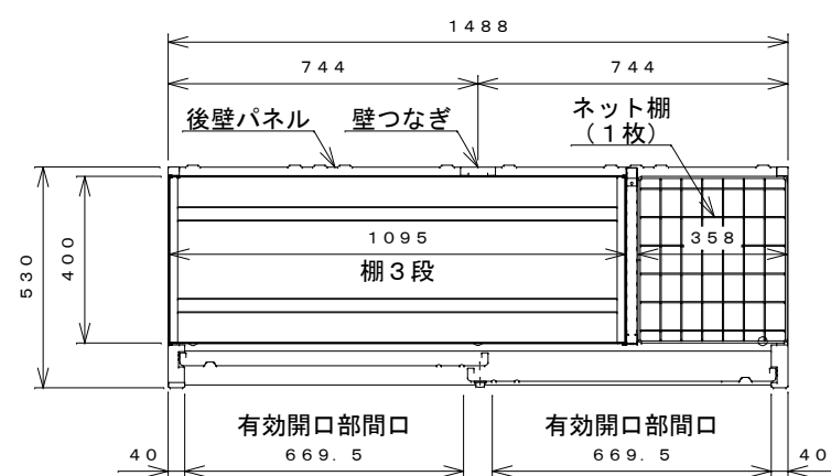
平面断面图
