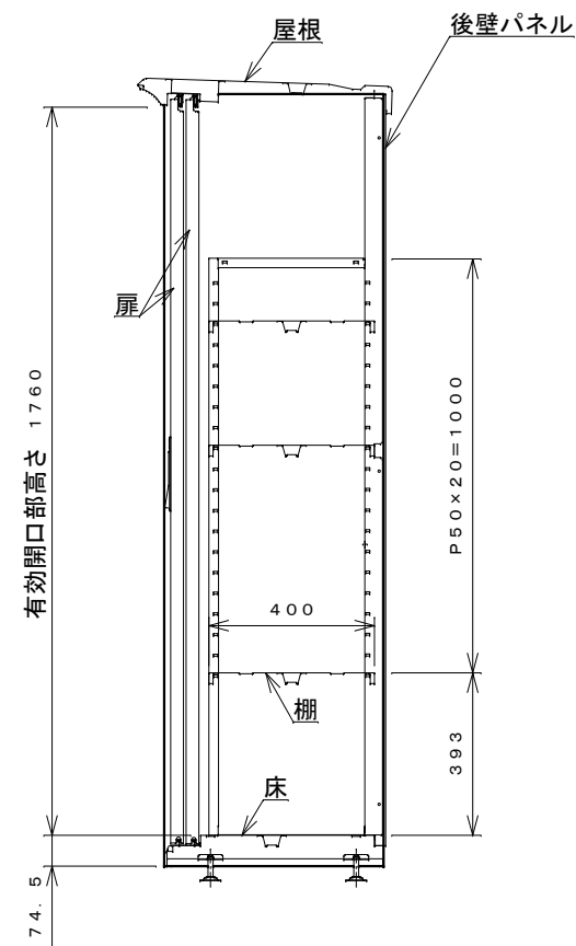
側面断面図
