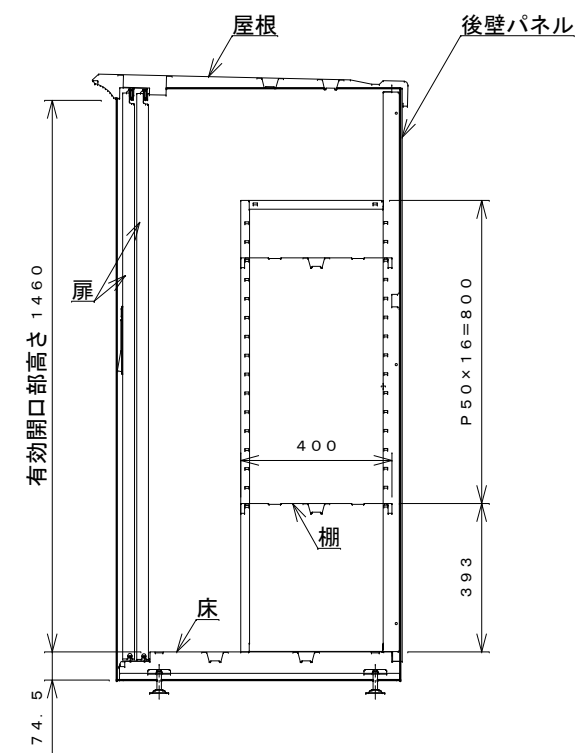
側面断面図
