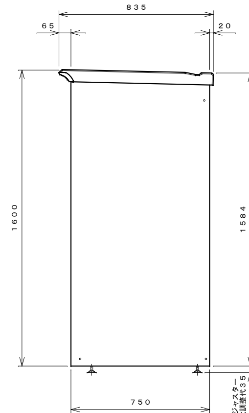
右側面図
