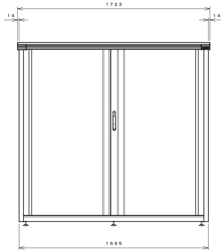
正面図
