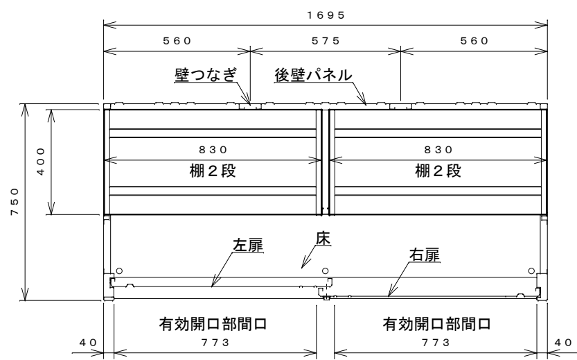
平面断面図
