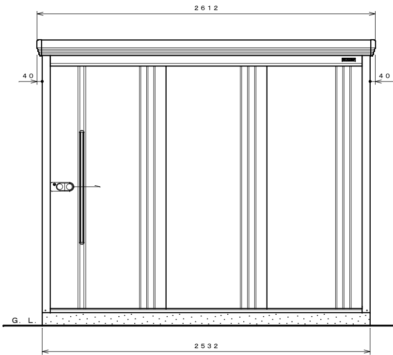
正面図 S=1:20
