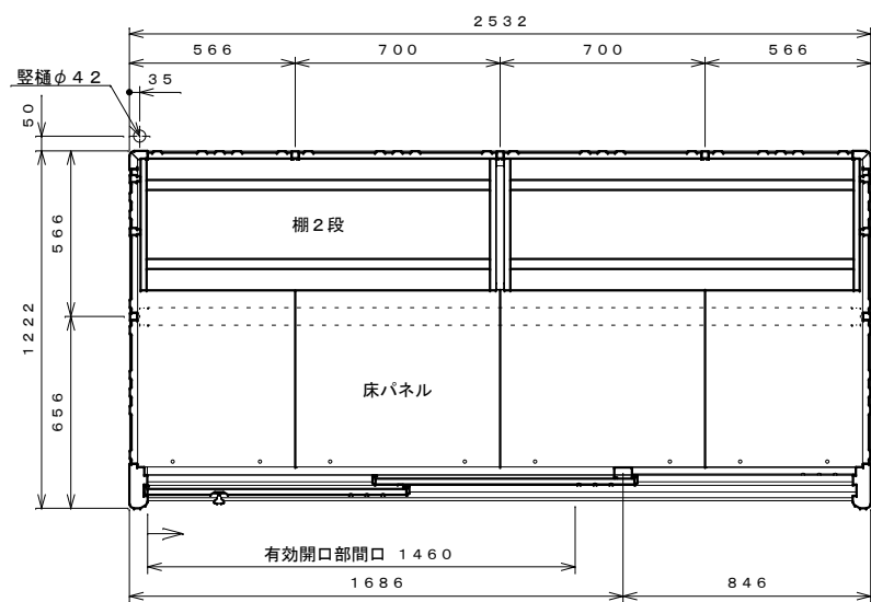
平面図 S=1:20
