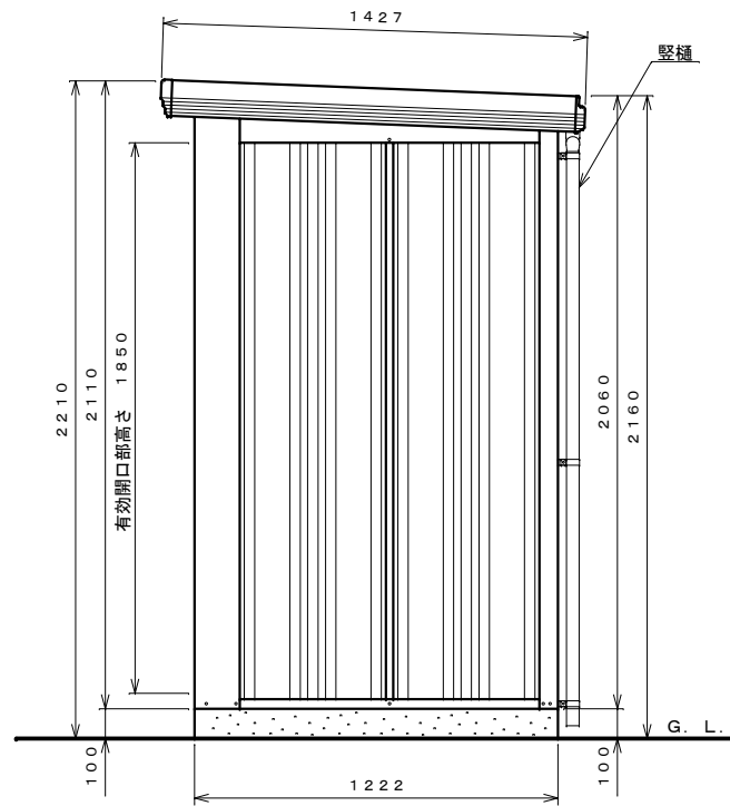
側面図 S=1:20
