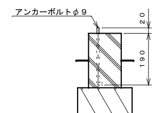
アンカーボルト埋設図 S=1:10
