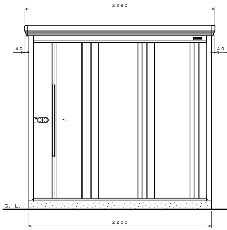
正面図 S=1:20
