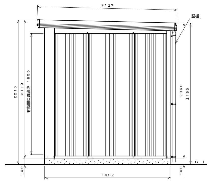
側面図 S=1:20
