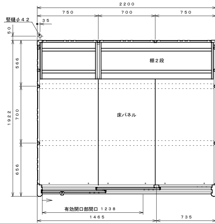
平面図 S=1:20
