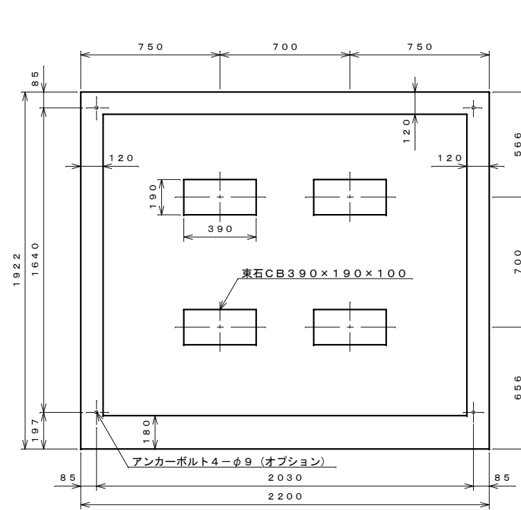
基礎伏せ図 S=1:20
