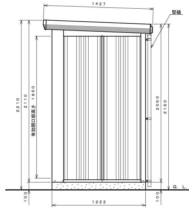
側面図 S=1:20
