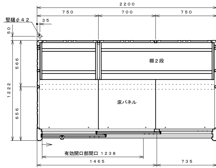
平面図 S=1:20
