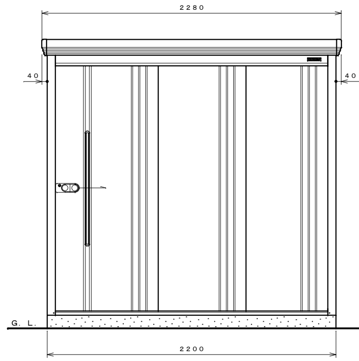
正面図 S=1:20
