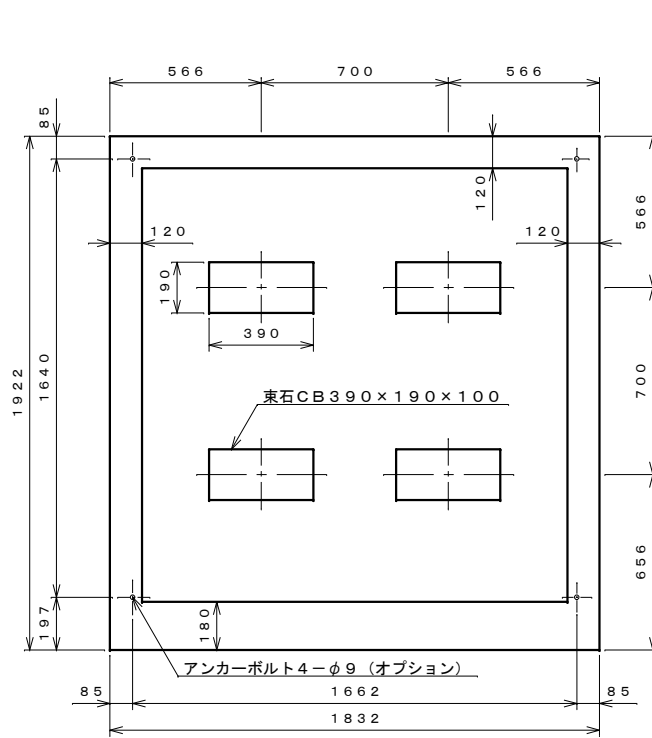
基礎伏せ図 S=1:20
