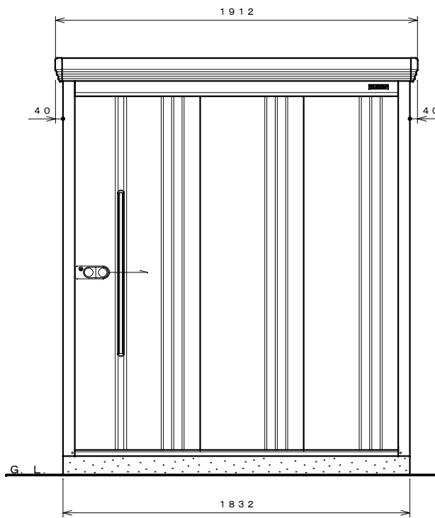
正面図 S=1:20
