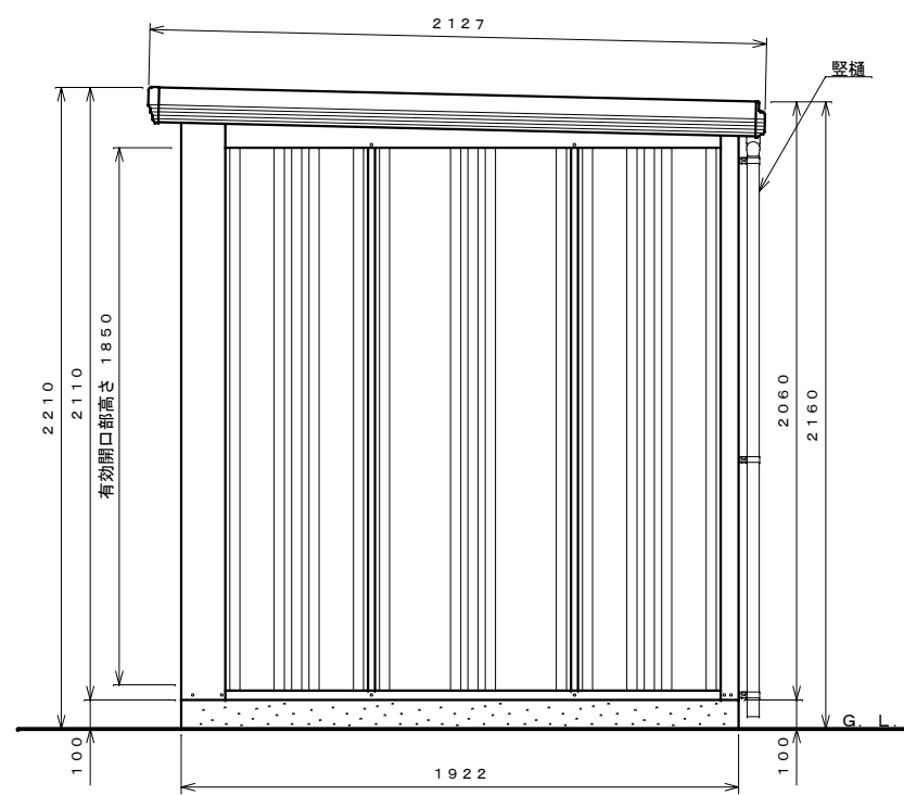
側面図 S=1:20
