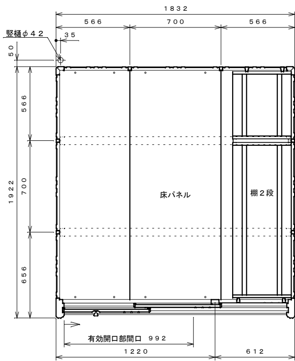
平面図 S=1:20
