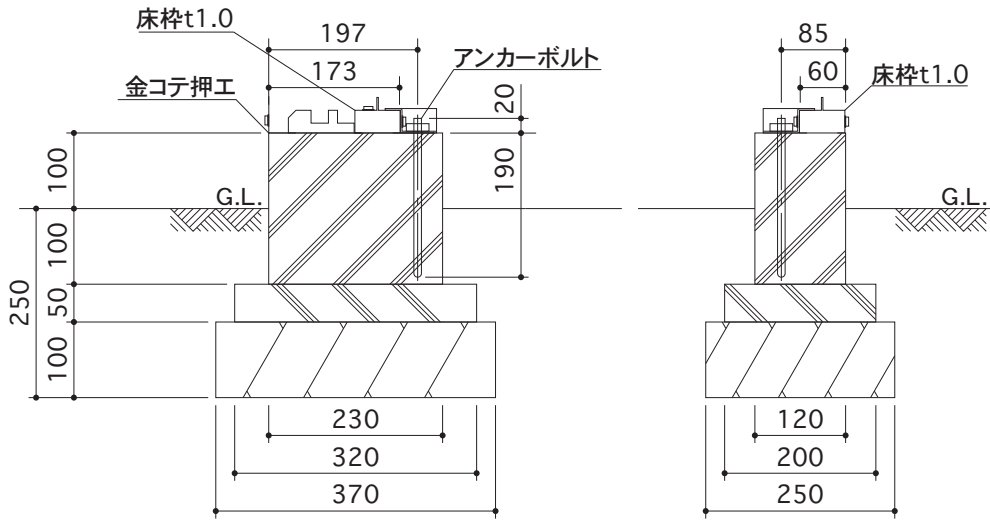
A-A断面図
