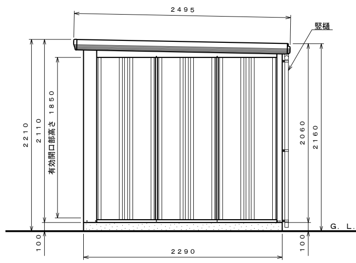
側面図 S=1:30
