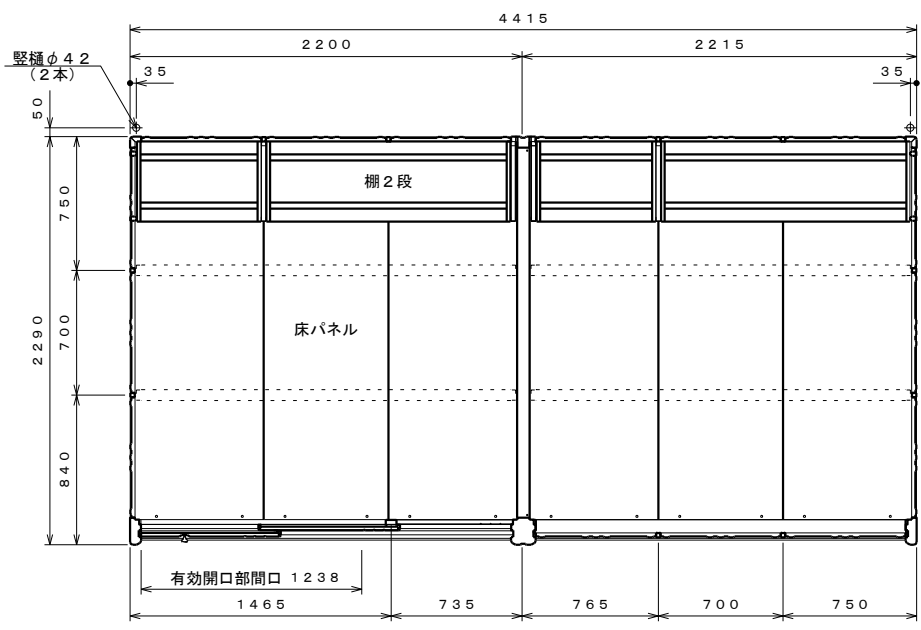
平面図 S=1:30
