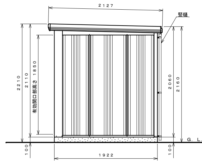
側面図 S=1:30
