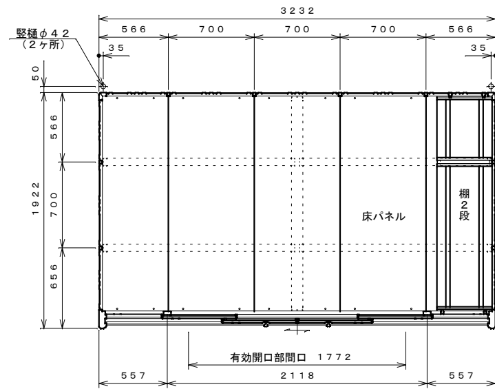
平面図 S=1:30
