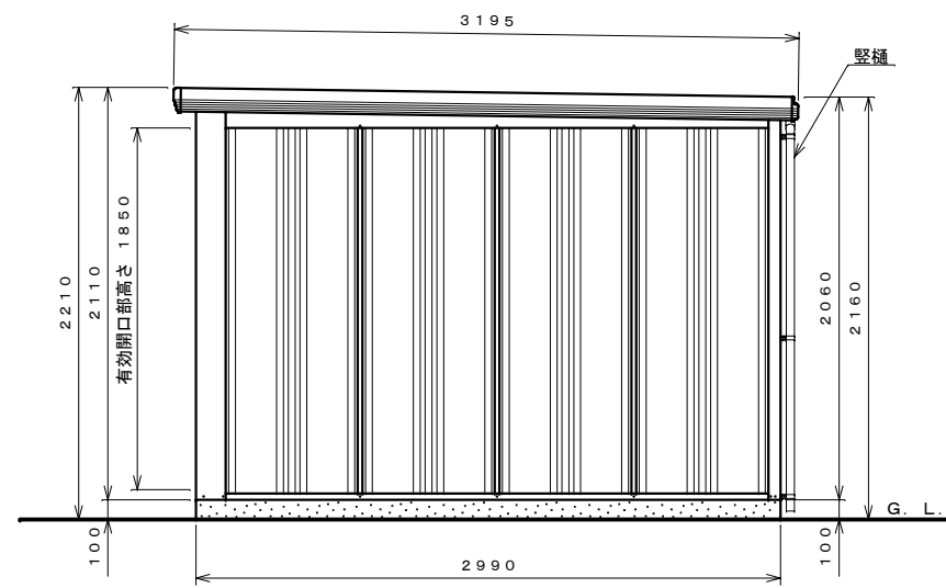
側面図 S=1:30
