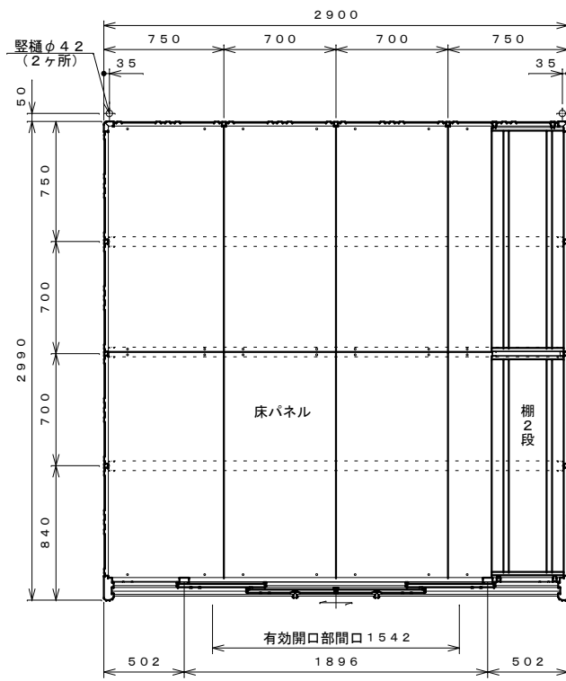
平面図 S=1:30
