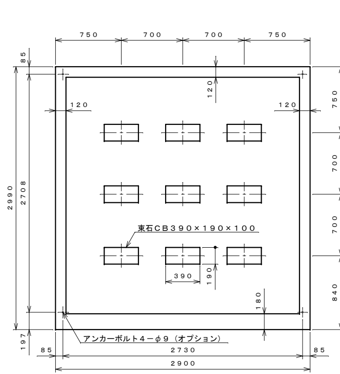
基礎伏せ図 S=1:30
