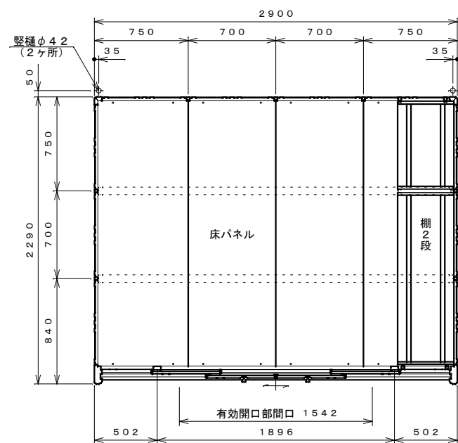
平面図 S=1:30
