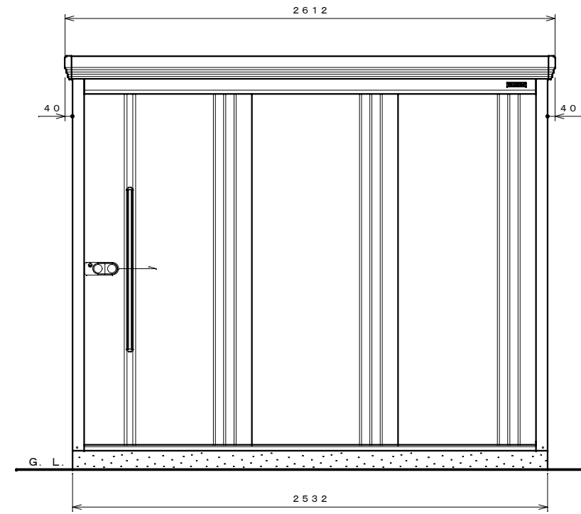
正面図 S=1:20
