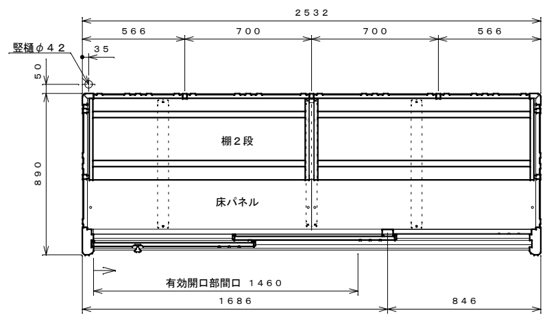
平面図 S=1:20
