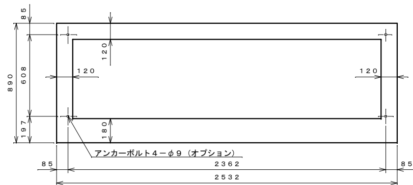
基礎伏せ図 S=1:20
