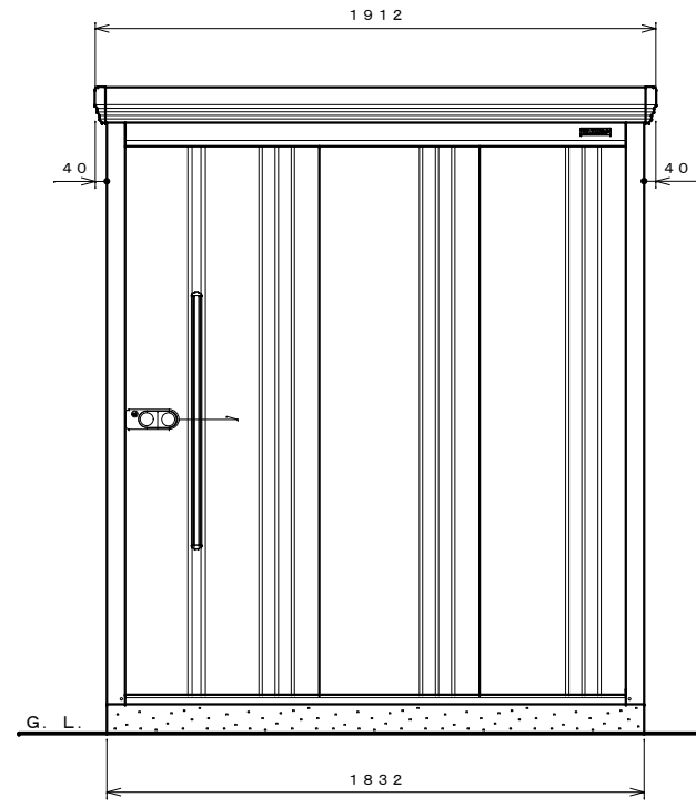
正面図 S=1:20
