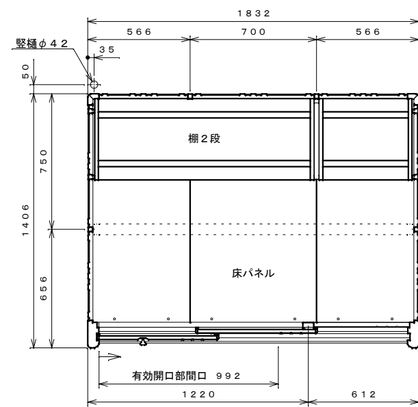
平面図 S=1:20
