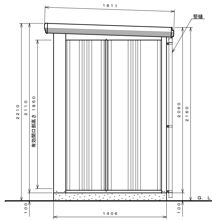
側面図 S=1:20
