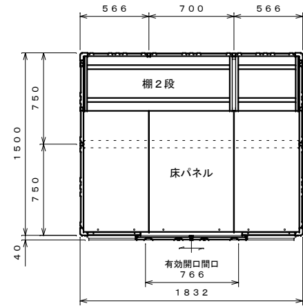
平面図 S=1:30
