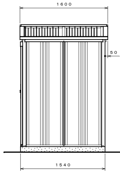
側面図 S=1:30
