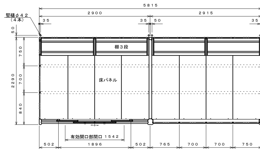
平面図 S=1:40
