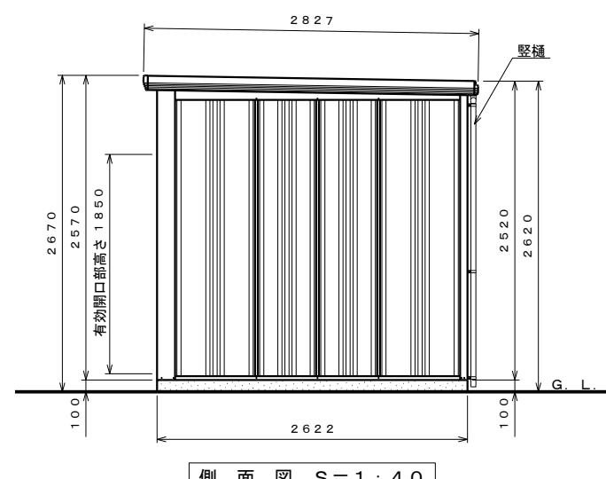
側面図 S=1:40
