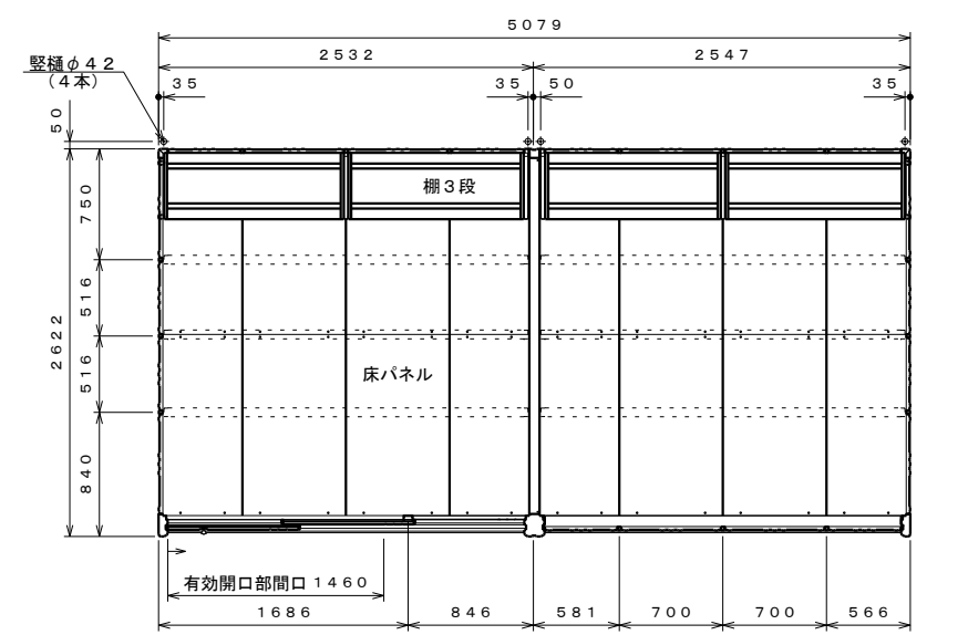
平面図 S=1:40
