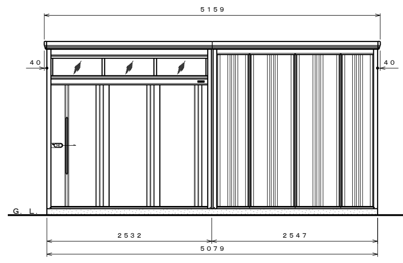
正面図 S=1:40
