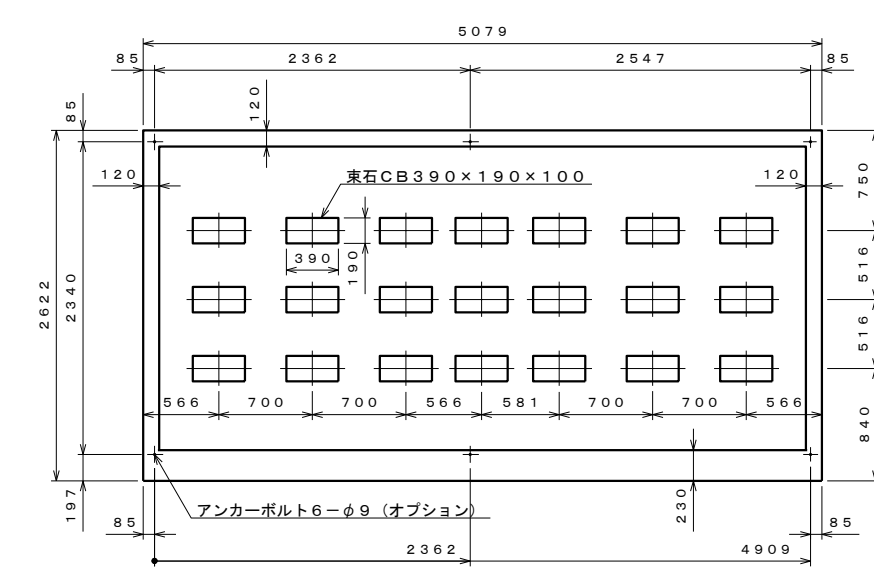
基礎伏せ図 S=1:40
