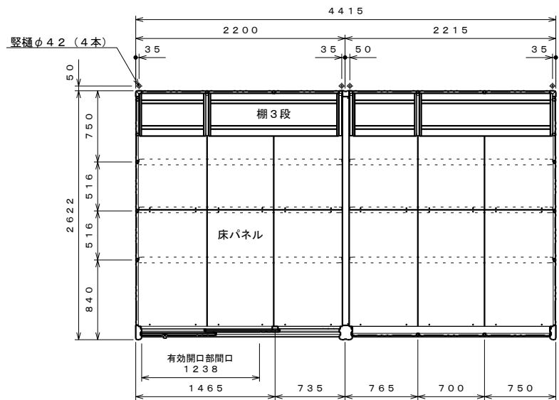
平面図 S=1:40
