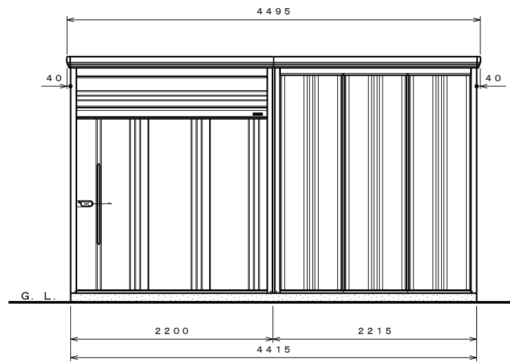
正面図 S=1:40
