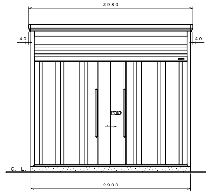
正面図 S=1:30
