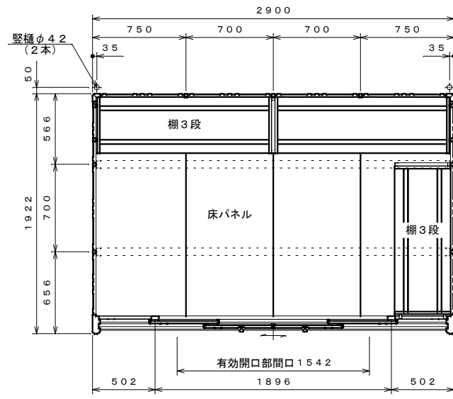
平面図 S=1:30
