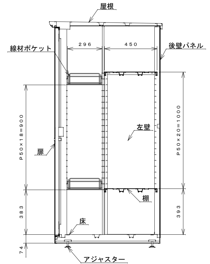
側面断面図
