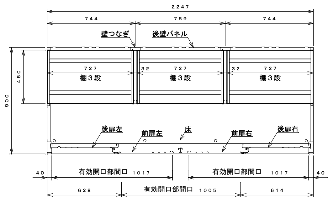
平面断面図
