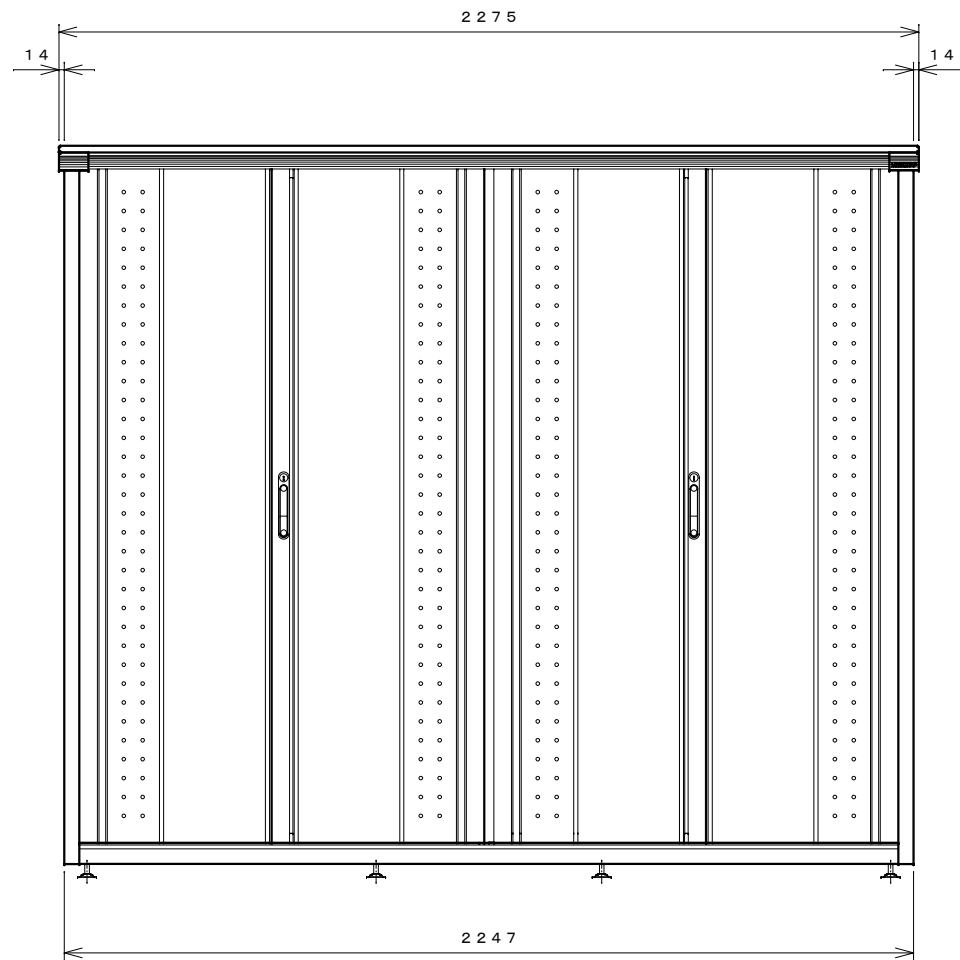
正面図
