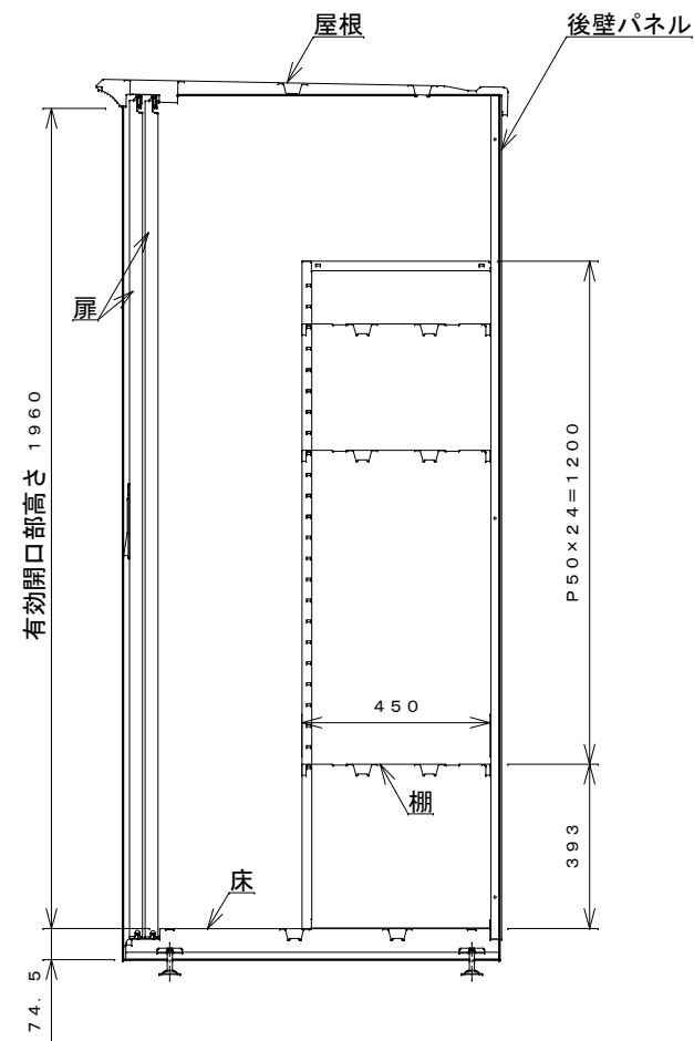
側面断面図
