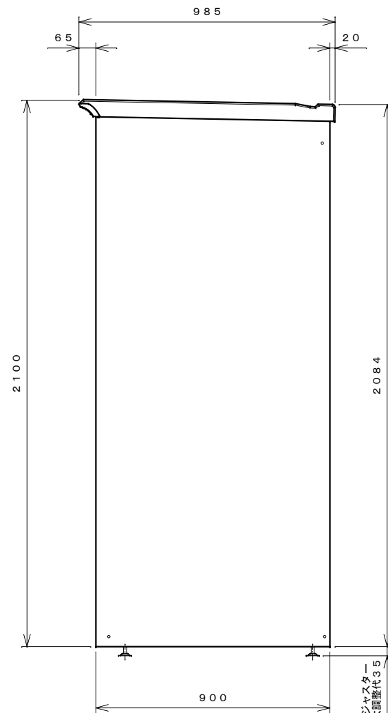
右側面図
