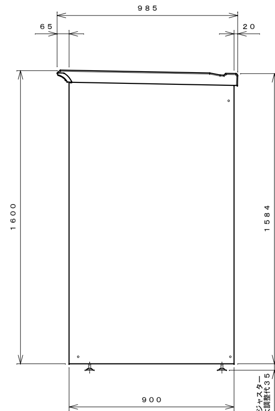
右側面図
