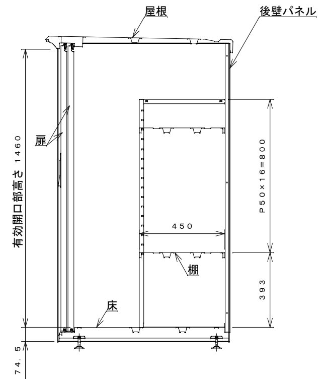
側面断面図
