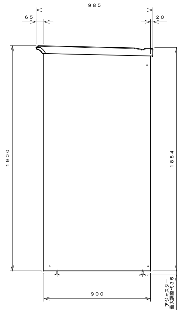
右側面図
