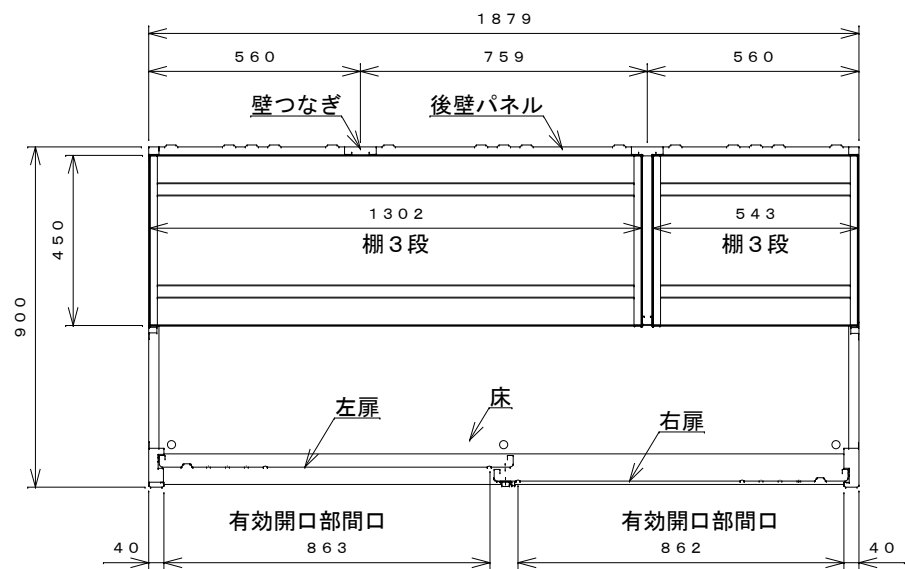
平面断面図
