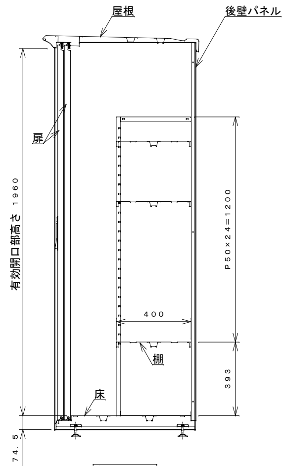
側面断面図
