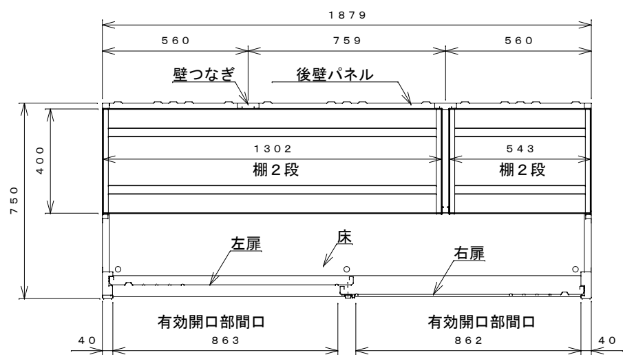
平面断面図
