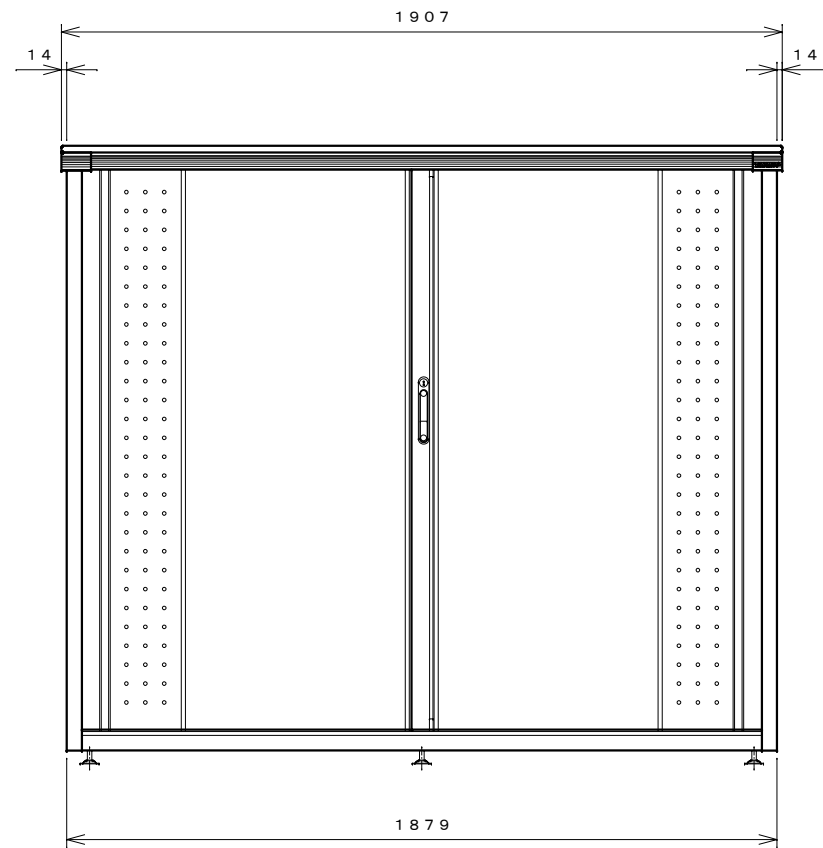
正面図
