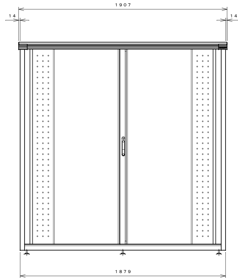
正面図
