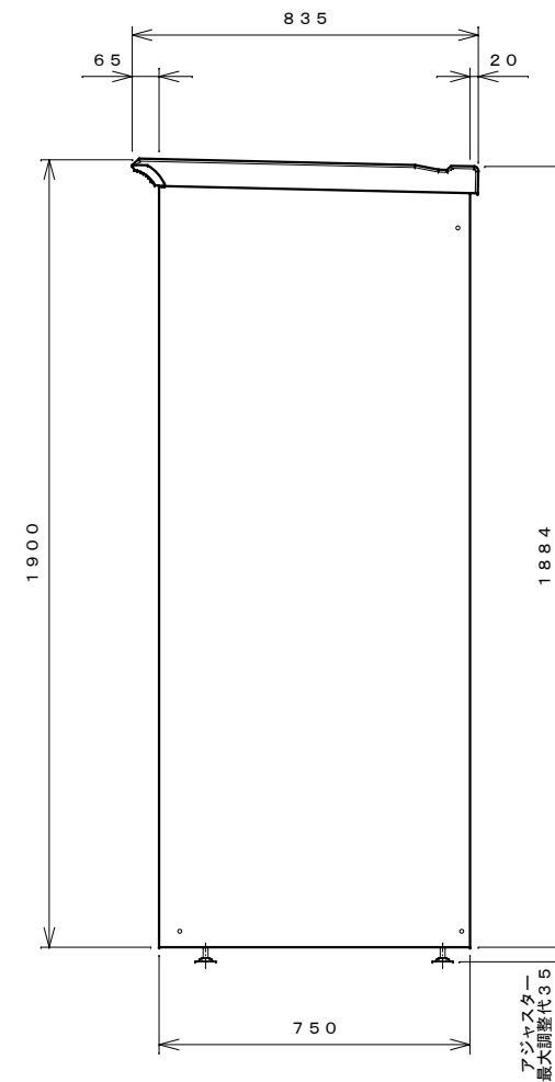
右側面図
