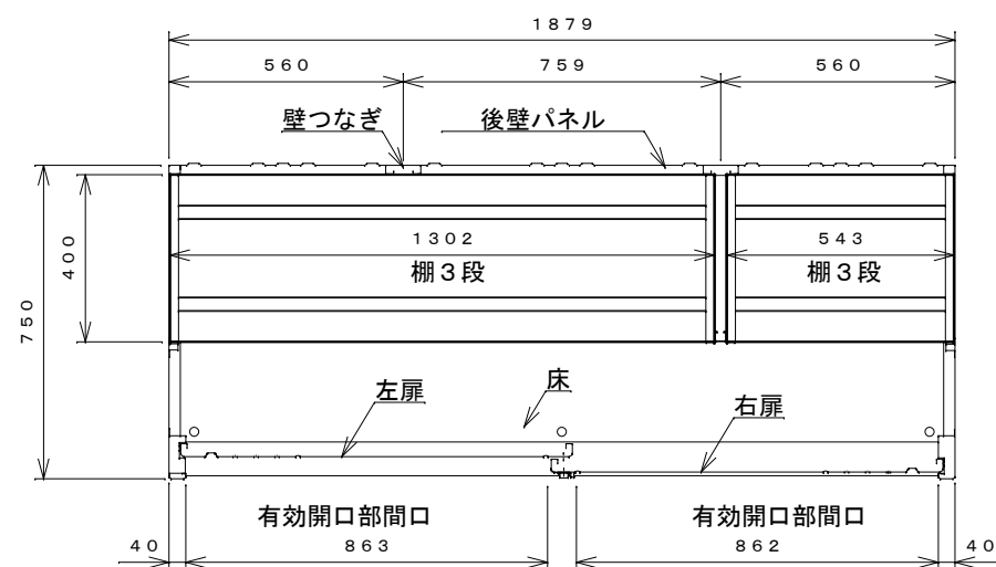
平面断面図
