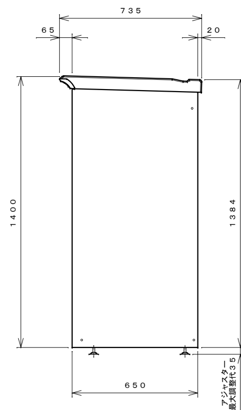
右側面図
