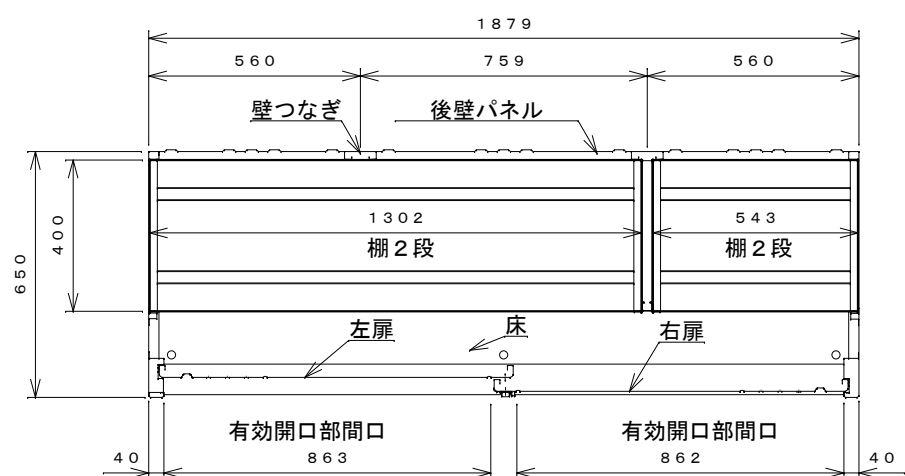
平面断面図
