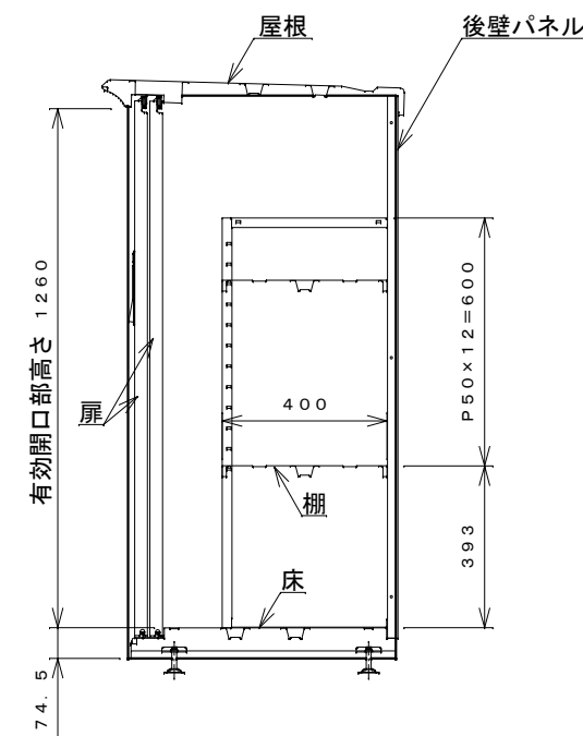
側面断面図
