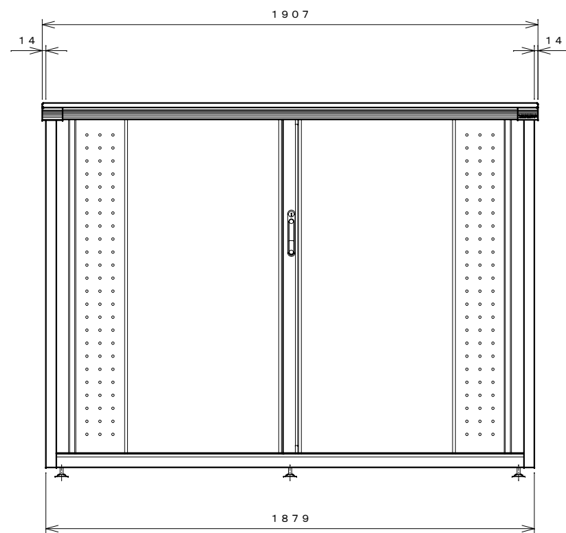
正面図
