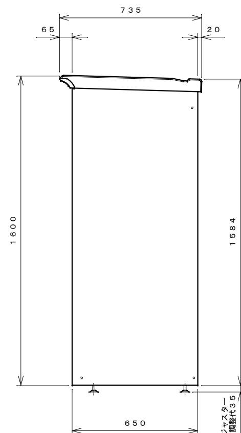
右側面図
