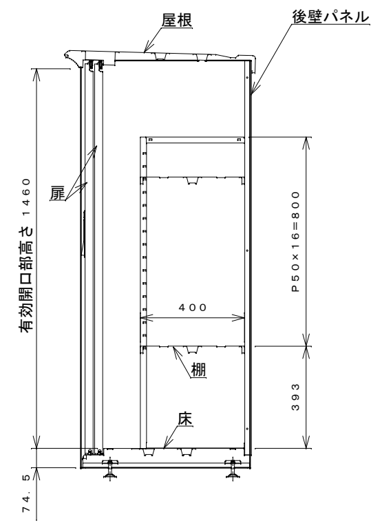
側面断面図
