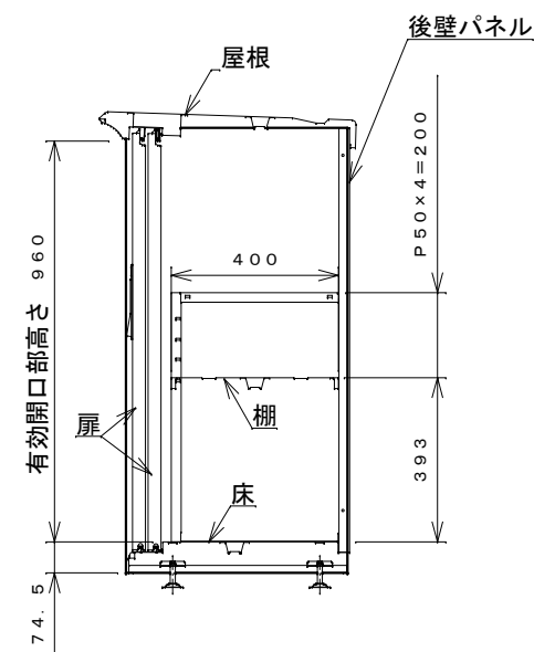
側面断面図
