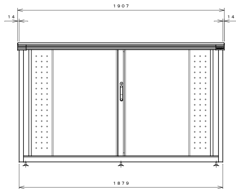
正面図
