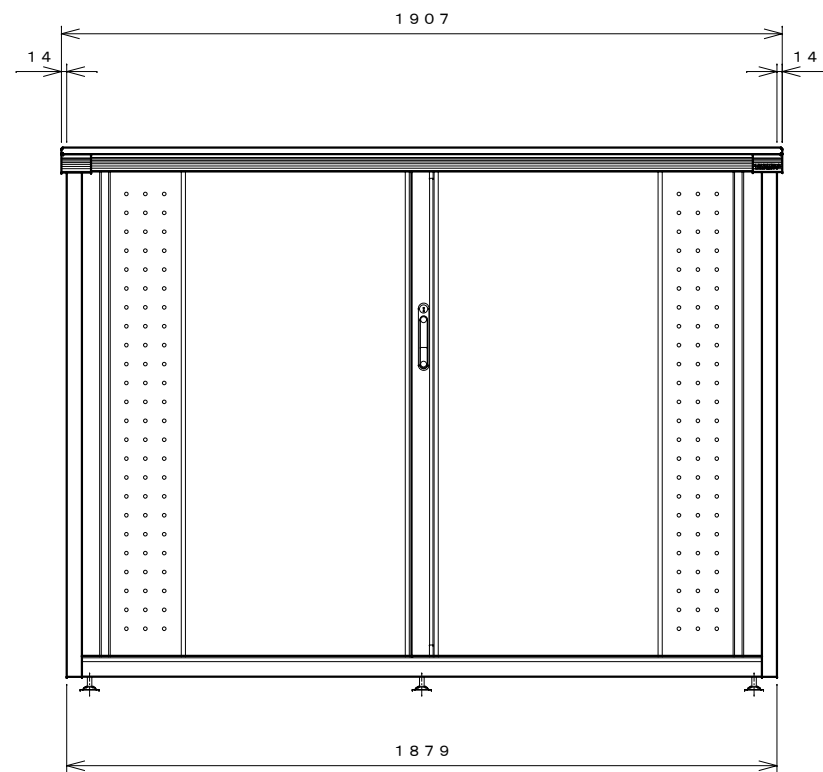
正面図
