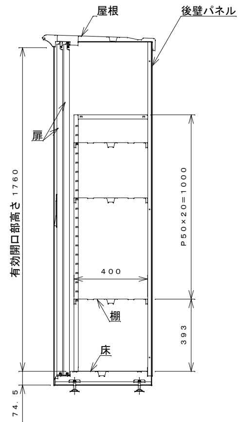
側面断面図
