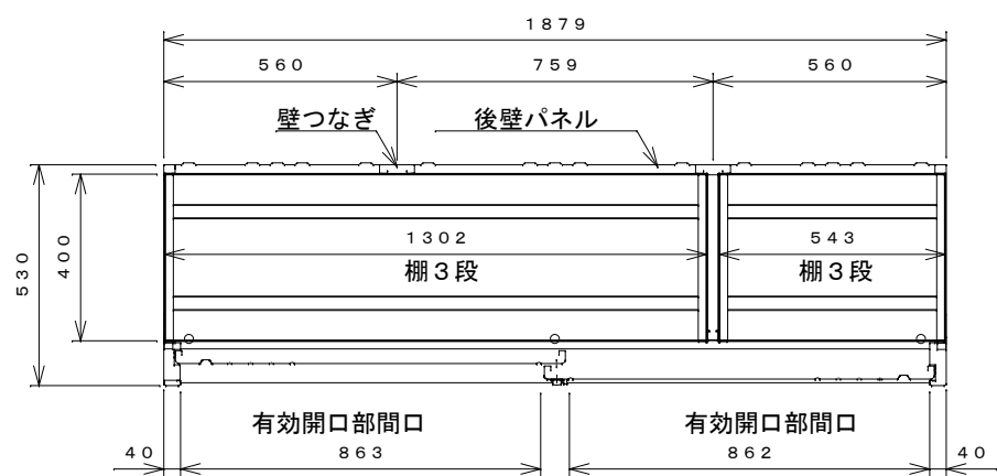
平面断面図
