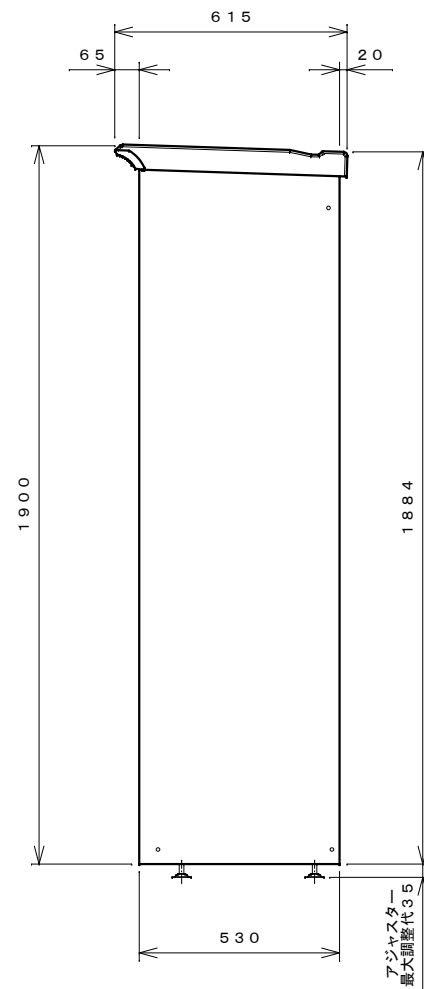
右側面図
