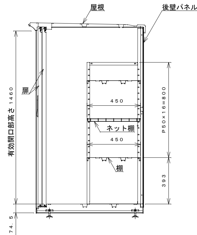
側面断面図
