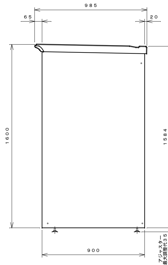
右側面図
