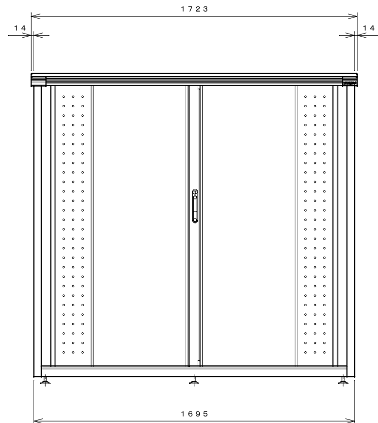
正面図
