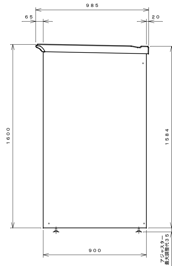
右側面図
