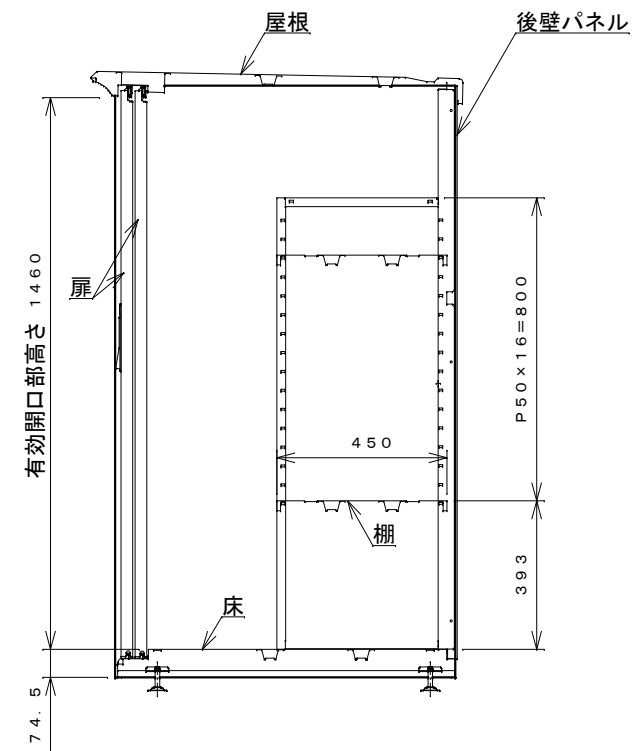
側面断面図
