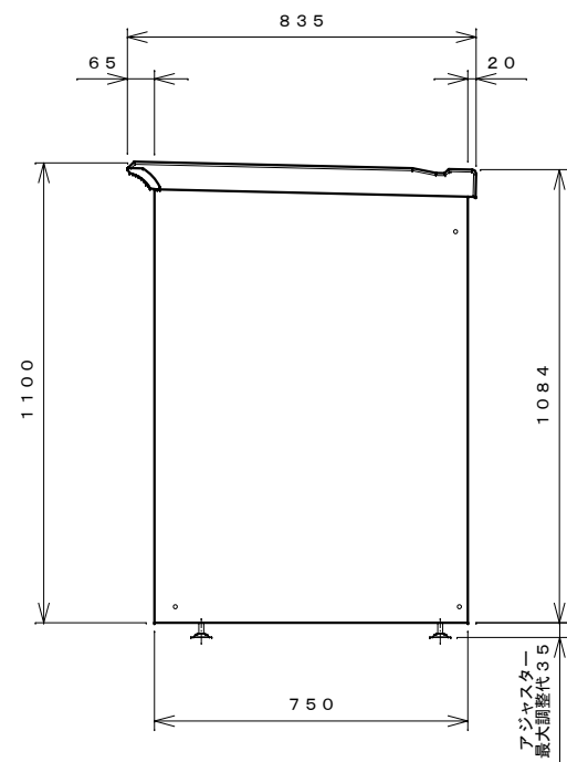
右側面図
