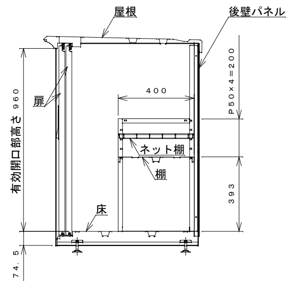
側面断面図
