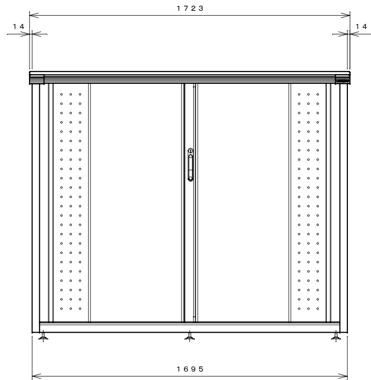
正面図
