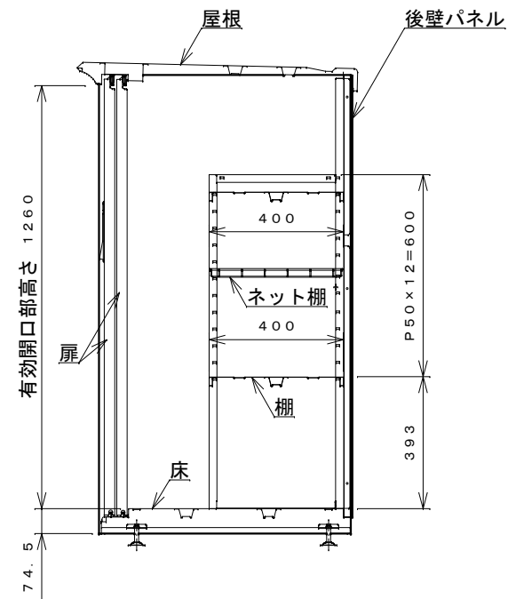
側面断面図
