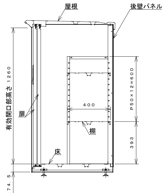
側面断面図
