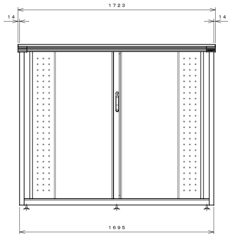
正面図
