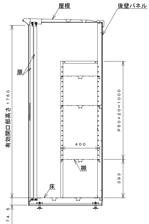
側面断面図
