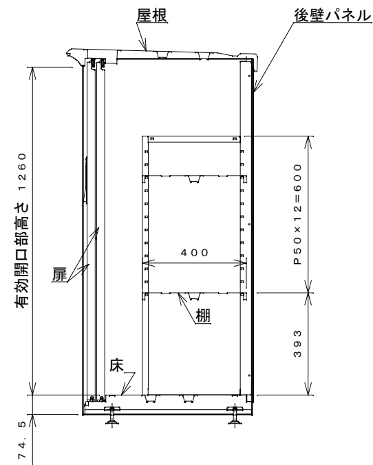
側面断面図
