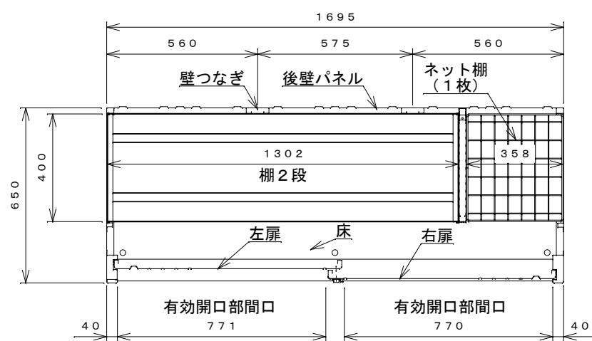
平面断面図
