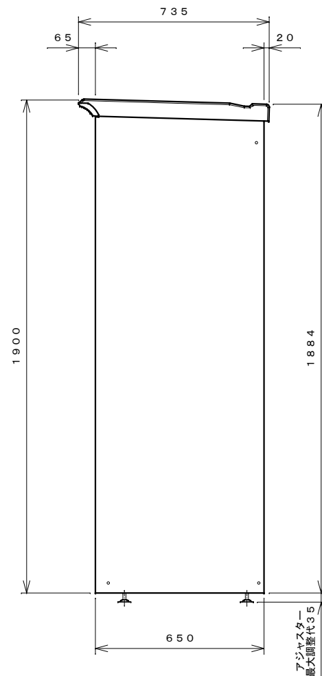
右側面図
