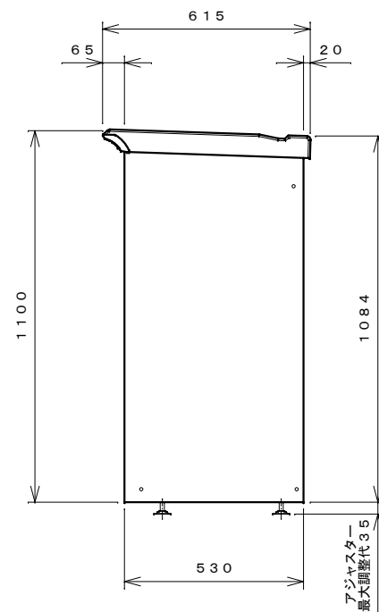
右側面図
