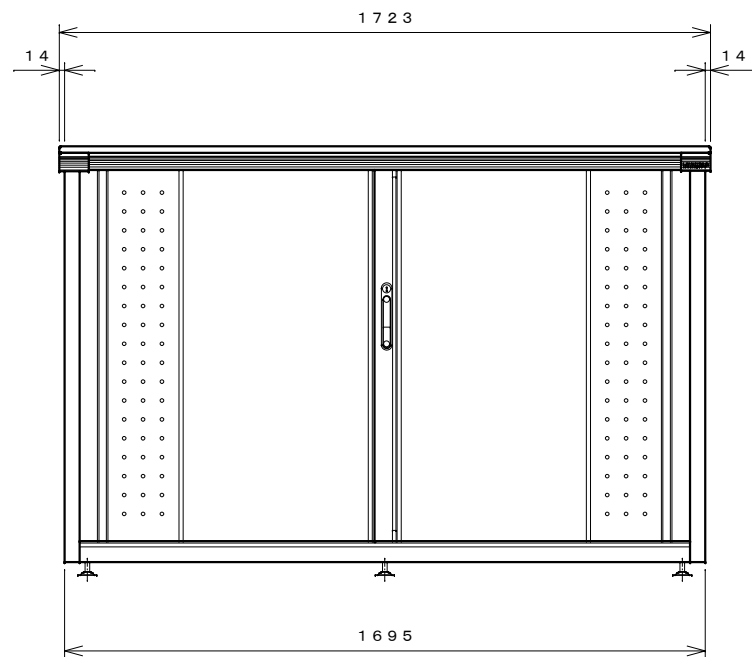
正面図
