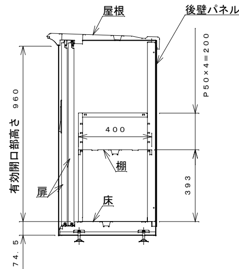
側面断面図
