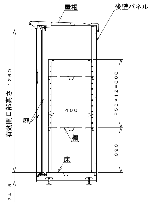
側面断面図
