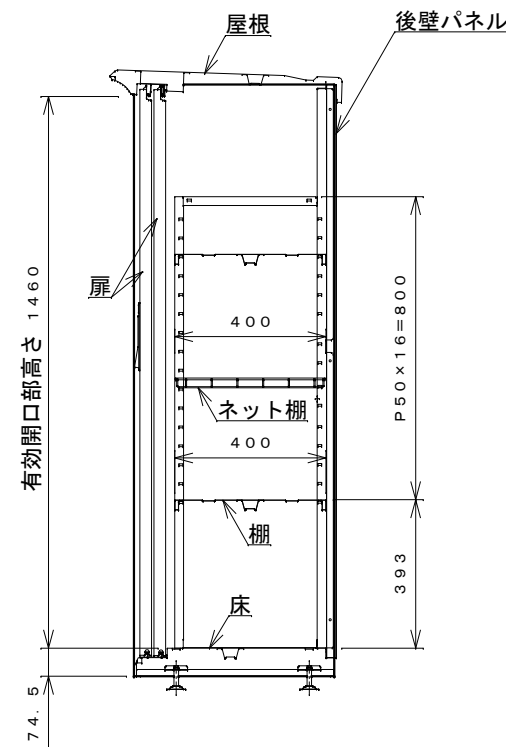
側面断面図
