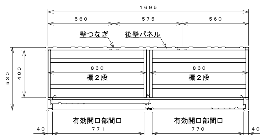
平面断面图
