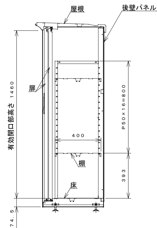
側面断面図
