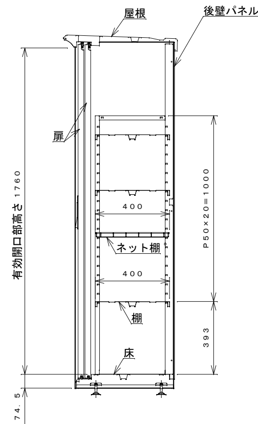
側面断面図
