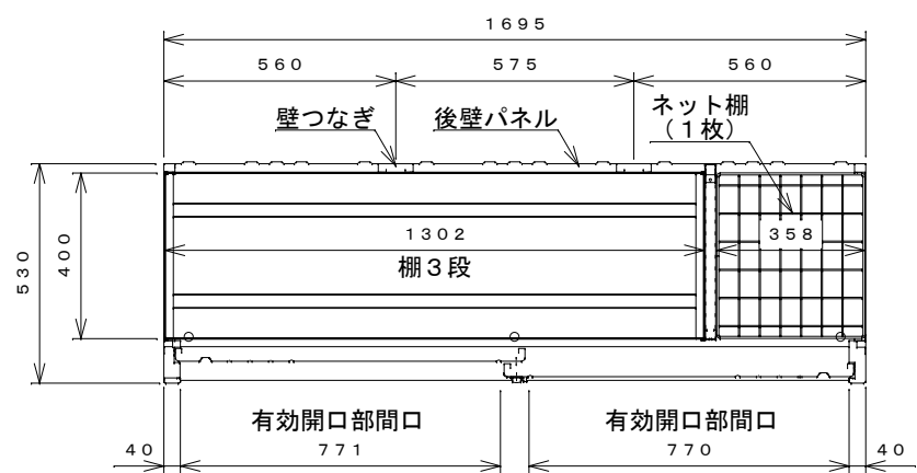
平面断面図
