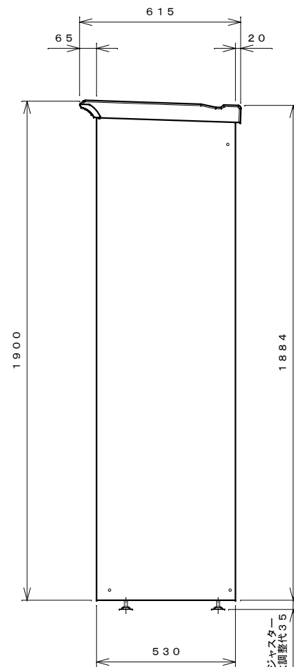
右側面図
