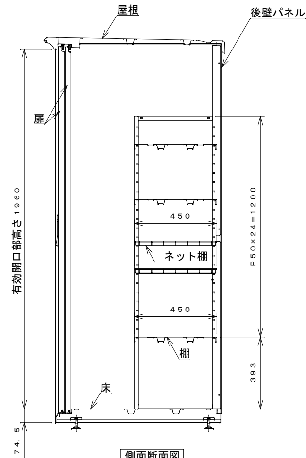
側面断面図
