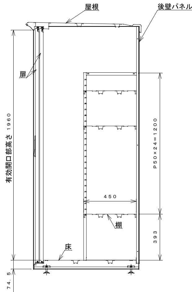
側面断面図
