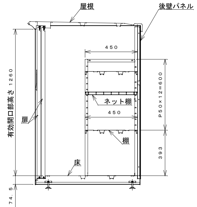
側面断面図
